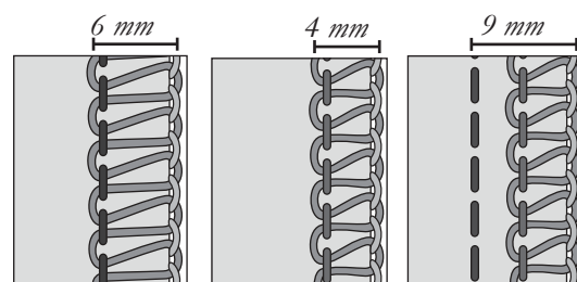
A) Vänster nål B) Höger nål C) Kedjesömnål
